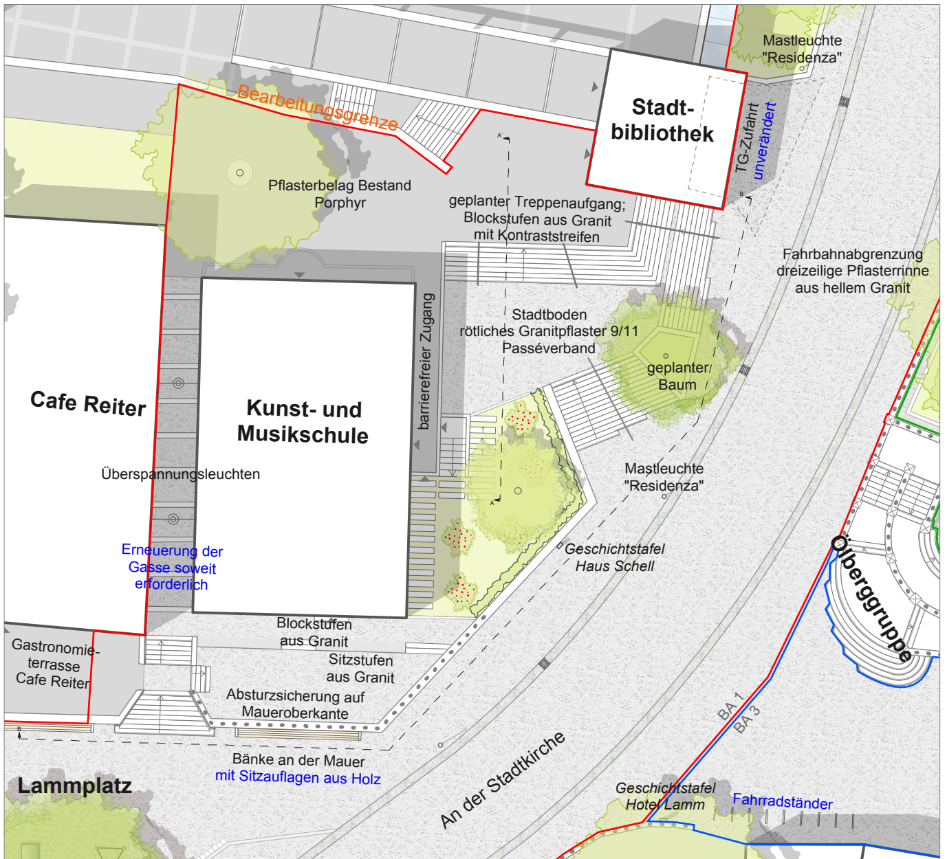
Lageplan neue Umgebung Kunst- und Musikschule
