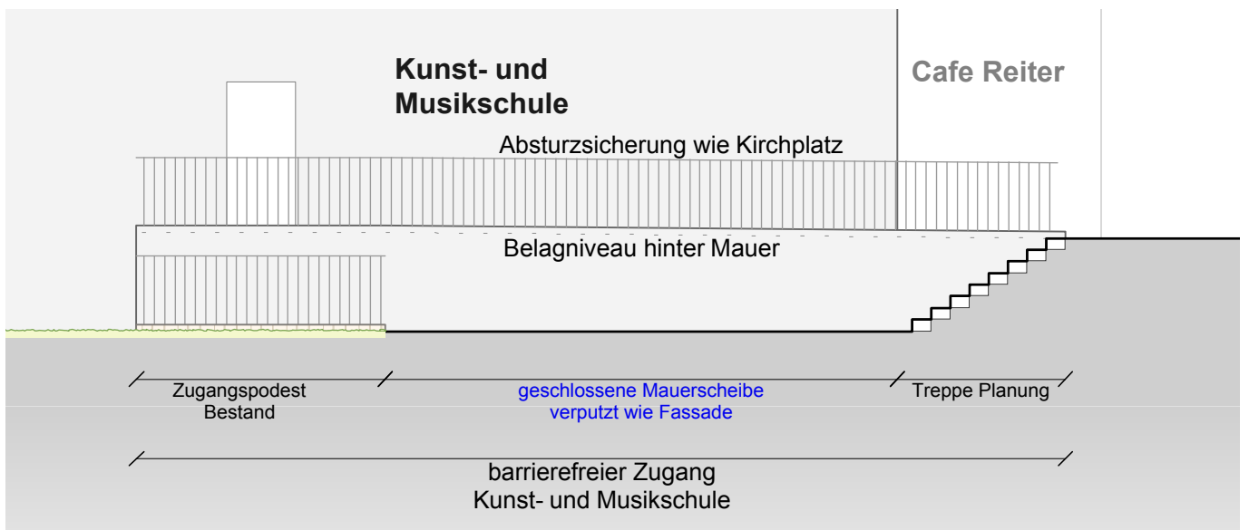
Ansicht des barrierefreien Zugangs zur Kunst- und Musikschule, Schnitt A - A'
