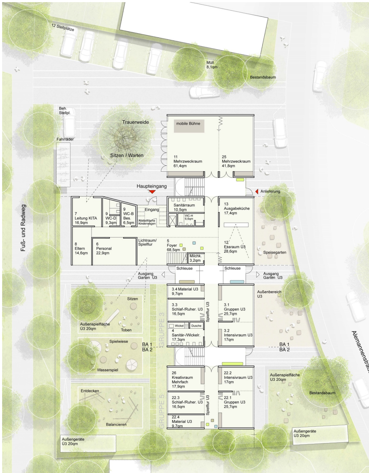
Erdgeschoss
