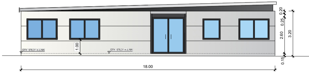
Ansicht Süd-West
