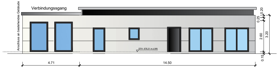
Ansicht Süd-Ost
