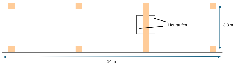
Vogelansicht
