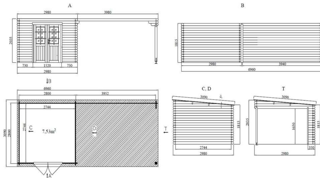
Grundriss Hühner- und Ziegenstall
